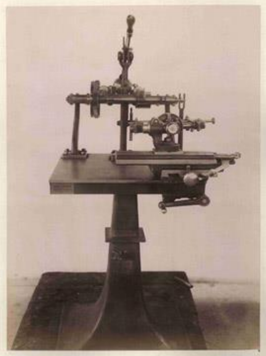
Machine à affûter les faises. (à la main) F 1
