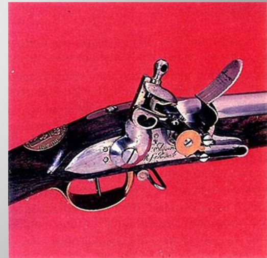
Platine avec bassinnet à Tambour montée sur le fusil des gardes du Corps du Roi modèle de 1816 2 ème type St-Étienne Manufacture Royale.
